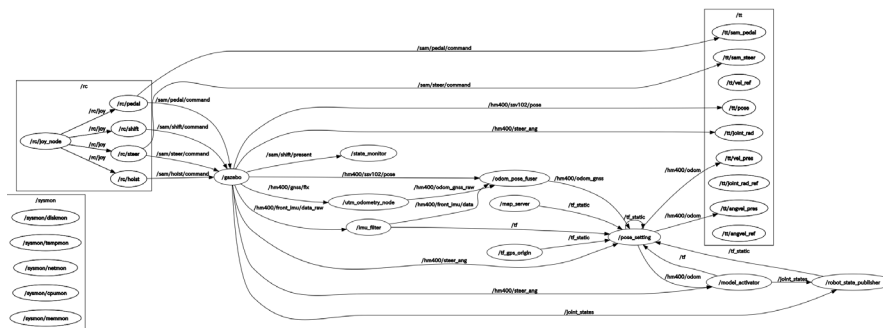
ソフトウェア構成(遠隔)
